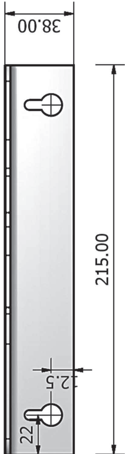
Figura 1. Plantilla para colocar los agujeros para los tornillos.
