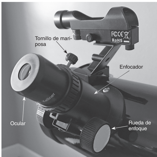
Figura 17. El ocular se muestra montado en el enfocador.
