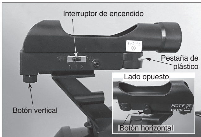
Figura 18. El telescopio buscador de punto rojo tiene botones de ajuste vertical y horizontal (insertado) para alinearlo con el telescopio.
