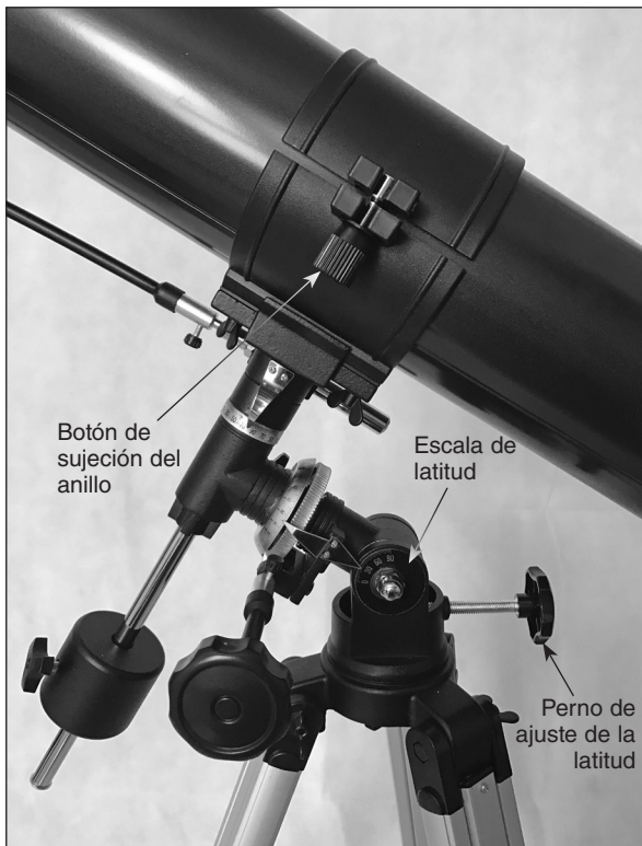
Figura 15. Coloque el tubo óptico en el anillo de tubo abierto, luego cierre el anillo y fíjelo con el botón de sujeción del anillo de tubo.
